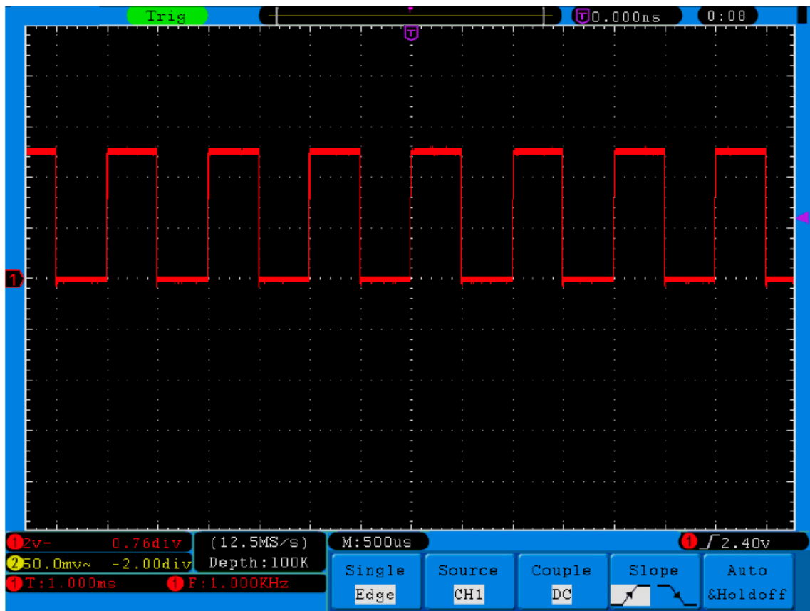
Fig.4-7 Auto set
